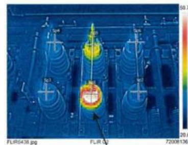
熱画像診断(サーモグラフィー)
