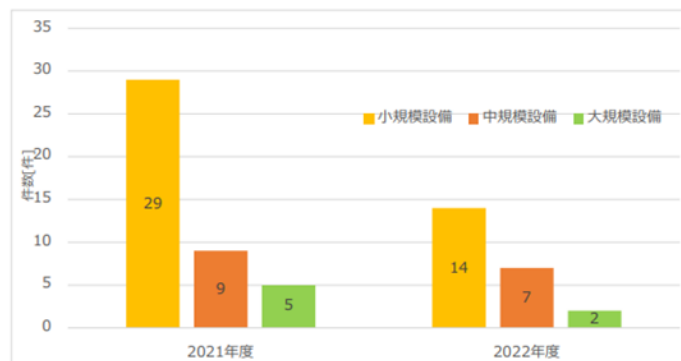
【図 3】 積雪による太陽電池発電設備の破損事故件数
